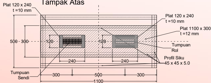
Gambar 21 Abutmen untuk Pengujian Jembatan
