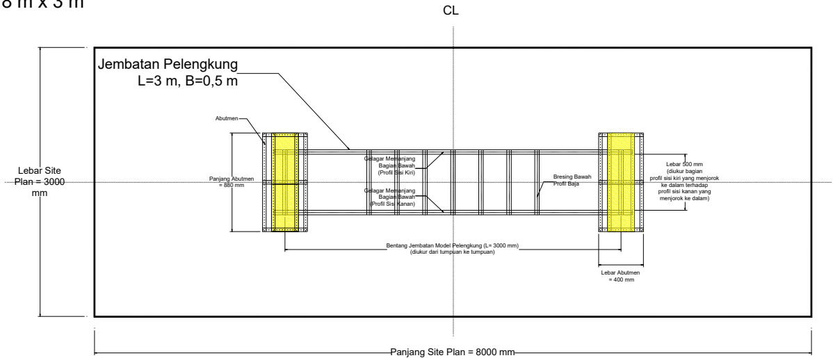
Gambar 17 Site Plan Tempat Perakitan Jembatan Model Pelengkung
