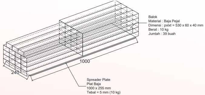
Gambar 11 Beban 400 kg Untuk Pengujian Jembatan Rangka Baja
