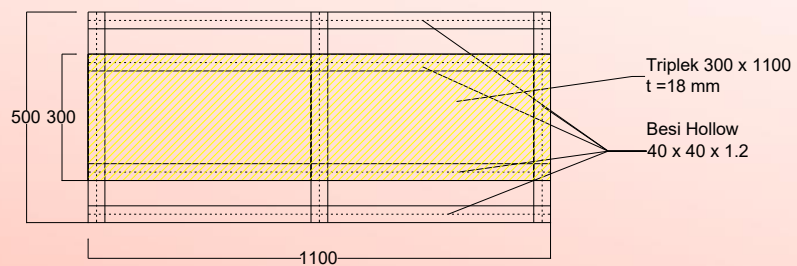
Gambar 23 Abutmen untuk display/perakitan Jembatan
