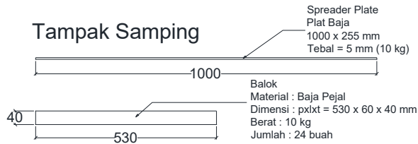
Gambar 26 Beban Untuk Pengujian Jembatan Model Pelengkung
